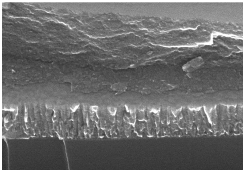
Рисунок 1.3 – Плотная структура W_4C толщиной 500 нм, полученная при температуре 50 °С, давлении Ar 0,16 Па и ионном ассистировании
